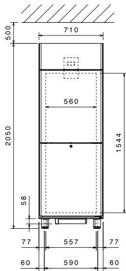
Front aanzicht
